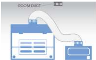
モード2 ヒューム排気ファンへ接続
