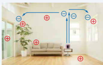
マイナス電子拡散イメージ図
