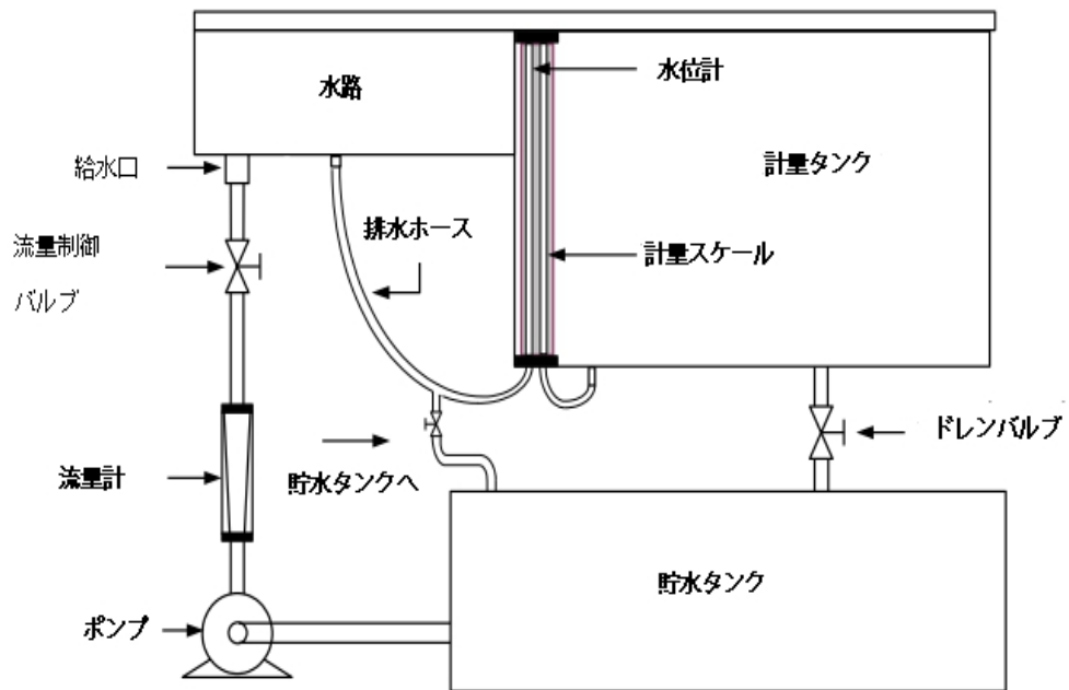
図1.b 配管図
